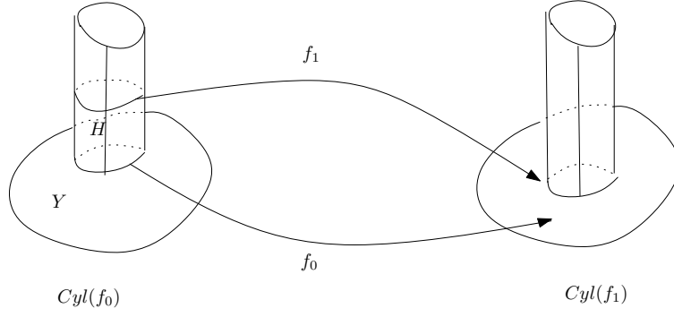
FIGURE 2 – L'application Cyl(f_0) \rightarrow Cyl(f_1) déduite de l'homotopie H .
