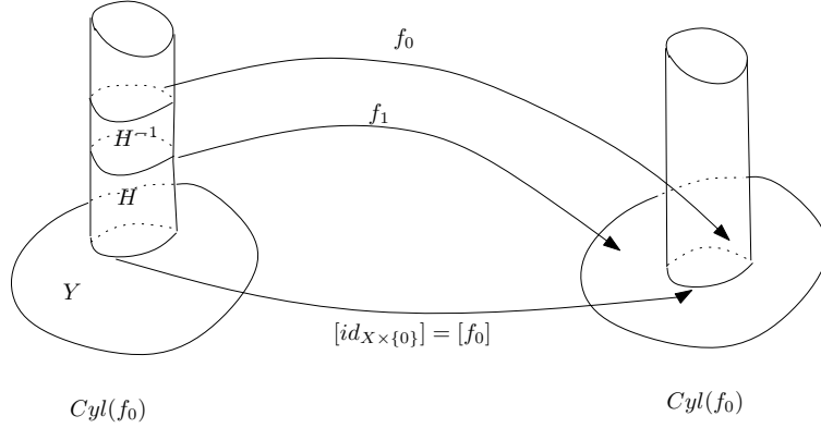
FIGURE 3 – L'équivalence d'homotopie K : Cyl(f_0) \rightarrow Cyl(f_0) déduite de l'homotopie H .
