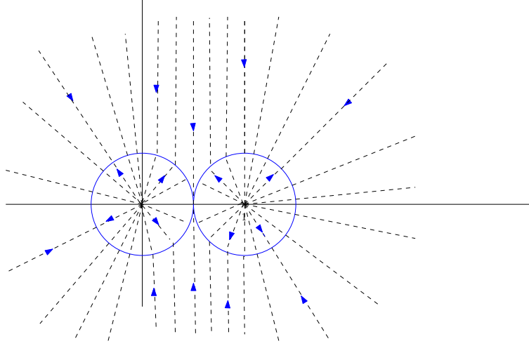
FIGURE 5 – La rétraction de \mathbb{C} \setminus \{0, 1\} sur la figure 8.
