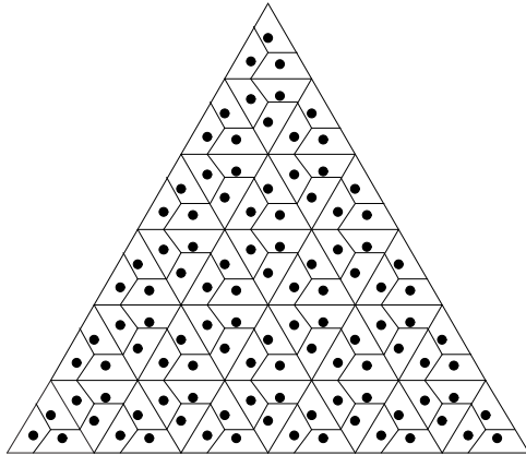
FIG. 6. Une décomposition simpliciale du quartier relativement à un domaine fondamental pour l'action des correspondances de Hecke et une orbite de Hecke (points noirs)
