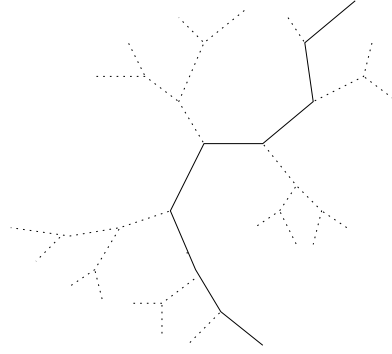
FIG. 12. Un appartement dans l'immeuble de \mathrm{PGL}_2 sur \mathbb{Q}_2 .
