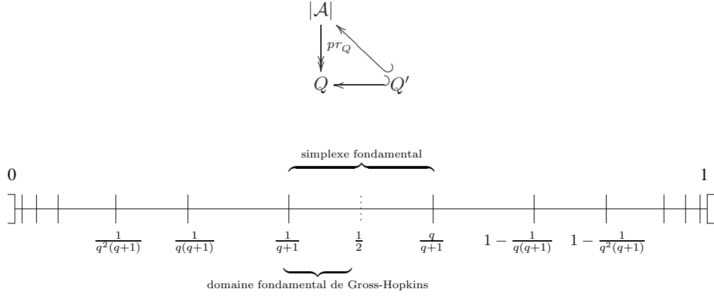
FIG. 8. La structure simpliciale de \Delta = ]0| dans le cas de GL_2
