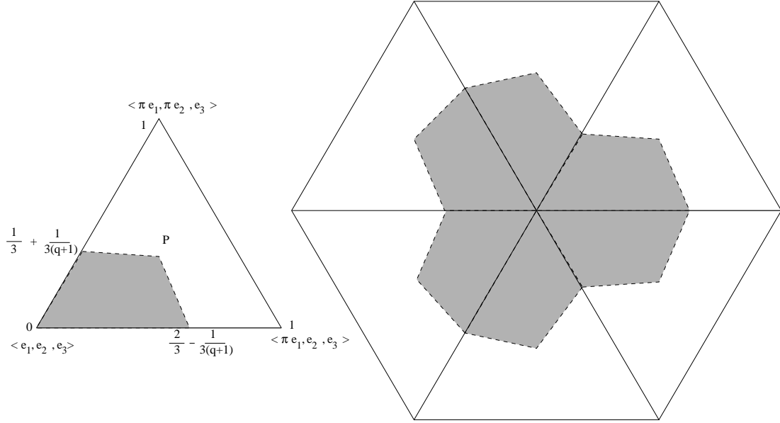
FIG. 7. L'image du domaine fondamental de Gross-Hopkins dans le "simplexe fondamental" du quartier et son image dans l'appartement
