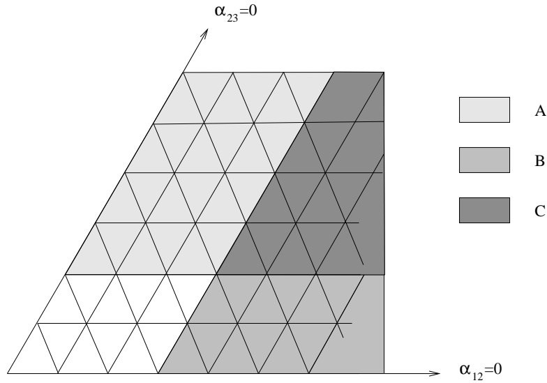
FIG. 5. Demi-appartement A = \exists sous-groupe canonique de rang 2 et niveau 3, B = \exists sous-groupe canonique de rang 1 et niveau 4, C = A \cap B
