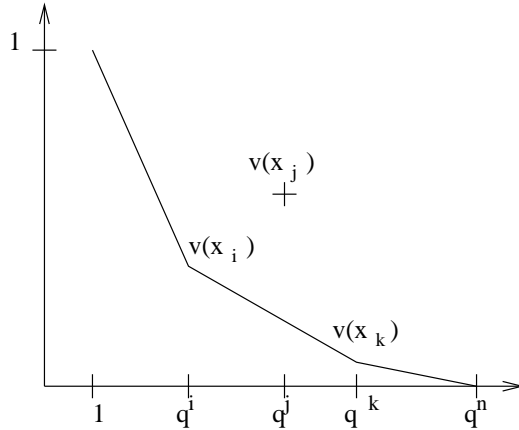
FIG. 2. Le polygone de Newton de la multiplication par \pi
