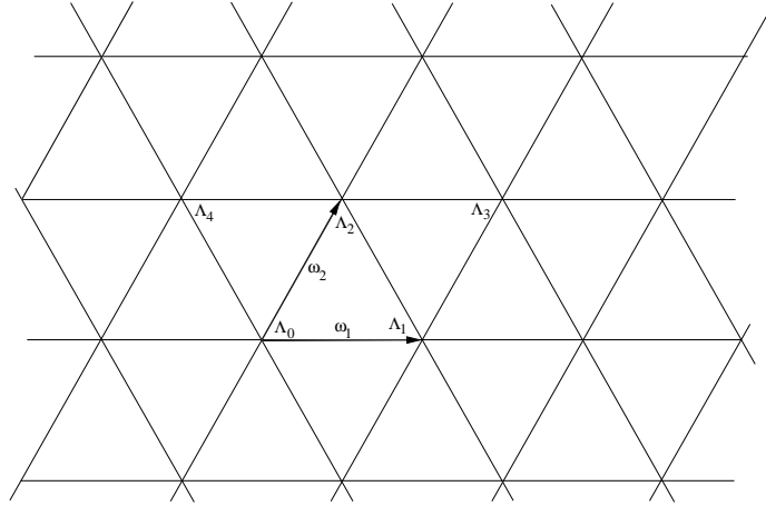
FIG. 14. Un appartement dans l'immeuble de \mathrm{PGL}_3
