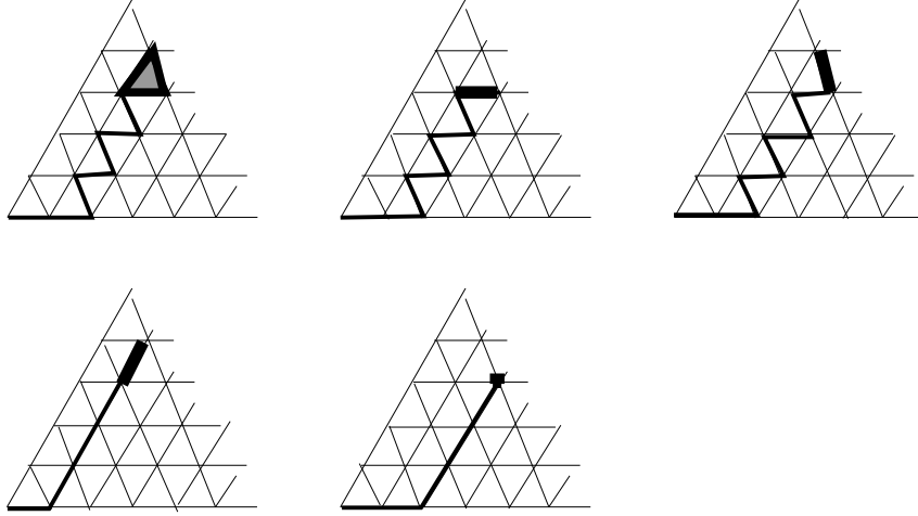
FIG. 3. Les cinq configurations possibles pour la filtration de ramification inférieure dans le cas de GL_3
