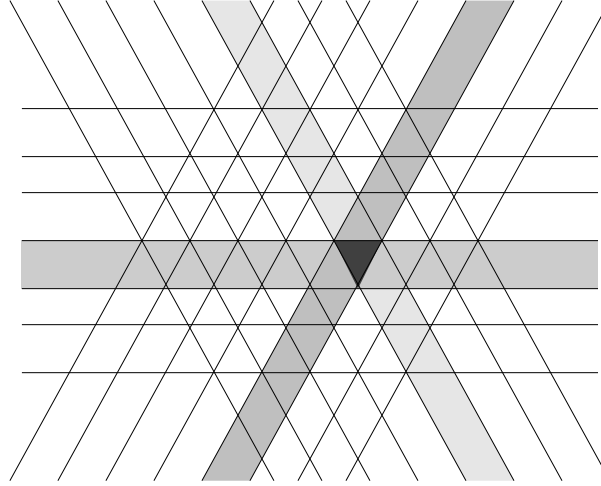
FIG. 15. Un simplexe paramétré par une intersection de demi-appartements
