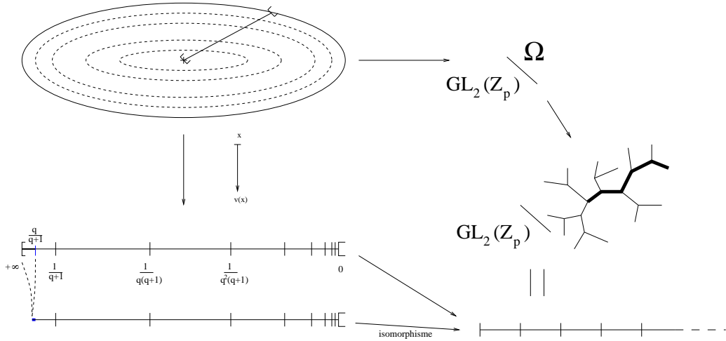
FIG. 1. Le cas de \mathrm{GL}_2
