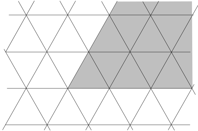
FIG. 16. Un quartier dans l'immeuble de \mathrm{PGL}_3
