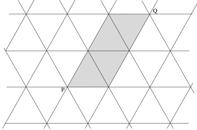
FIG. 17. L'enclos délimité par les points P et Q dans l'immeuble de \text{PGL}_3
