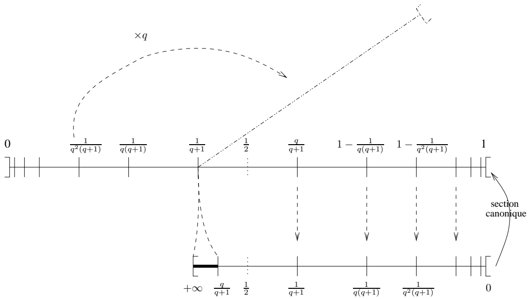
FIG. 9. L'application entre les squelettes de l'espace de Lubin-Tate en niveau Iwahori et celui sans niveau pour GL_2 (cette application est "multivaluée" en \frac{1}{q+1} ). La section canonique est définie sur le segment ]0, \frac{q}{q+1}[ d'image ]\frac{1}{q+1}, 1[ . L'opérateur de Hecke donné par l'élément non-trivial dans le normalisateur de l'Iwahori modulo l'Iwahori qui agit comme automorphisme de l'espace en niveau Iwahori correspond à la symétrie de centre \frac{1}{2} , x \mapsto 1 - x .
