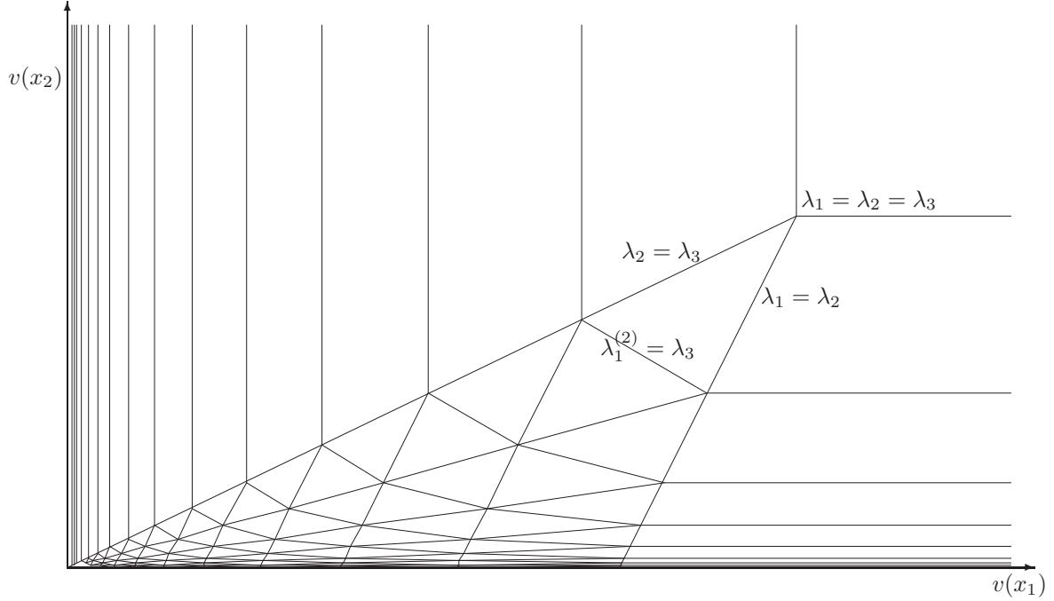
FIG. 4. La décomposition simpliciale de la boule p -adique ouverte de dimension 2
